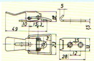
CL63222NI CHIUSURA A LEVA FERRO ZINCATO
